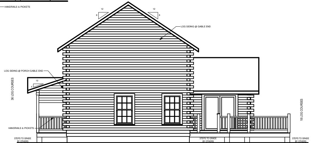
RIGHT ELEVATION
